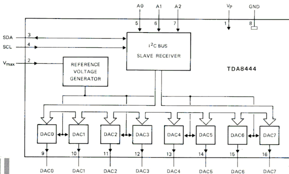
TDA 8444
