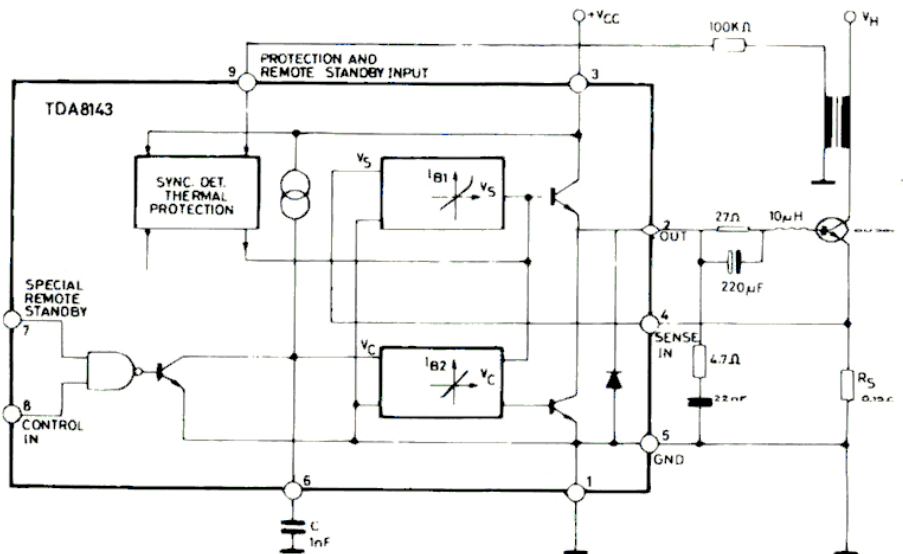
TDA 8143
